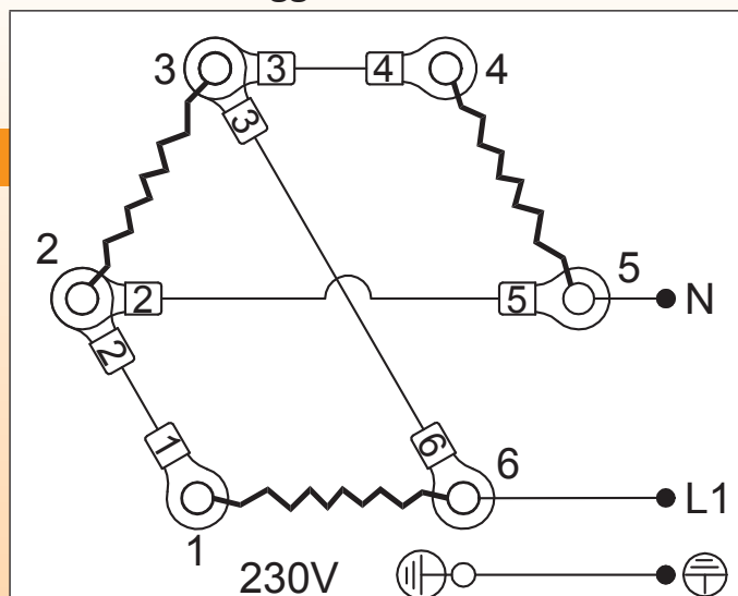
Posizione dei ponticelli in 220-240V monofase
