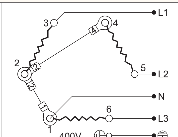
Posizione dei ponticelli in 380-400V 3 fasi
